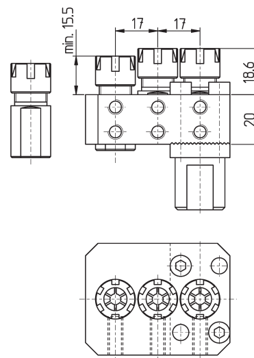
HVWP - CH3-17 mit 3 Einsätzen EM111620 with 3 Collet holders EM111620
