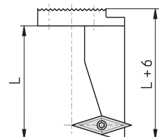
SVNCR11 (Ausführung rechts) (Version right)
