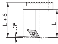
SDJCL07 (Ausführung links) (Version left)
