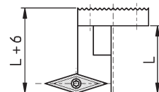
HVWPA-SVNCR11 (Ausführung rechts außen) (Version right external)
