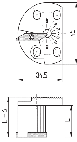
Ausführung links Version left
