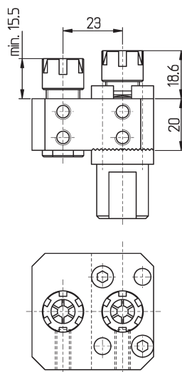
HVWP - CH2 mit 2 Einsätzen EM111620 with 2 Collet holders EM111620
