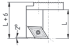
SDJCL11 (Ausführung links) (Version left)
