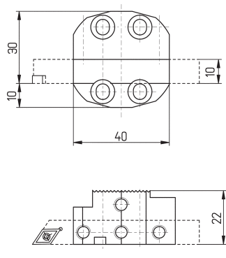
Bild 1 R + L + überkopf einsetzbar Useable r., l. + overhead
