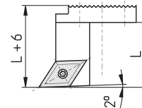
HVWPA-SDJCR11 (Ausführung rechts außen) (Version right external)
