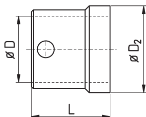
Anschlag - stopper
